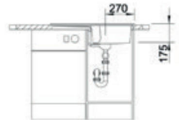
Ön Görünüm / Front View
