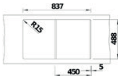
Tezgah Kesim Ölçüleri / Cut-Out
