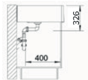
Tezgah Kesim Ölçüleri / Cut-Out
