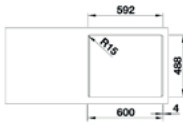
Tezgah Kesim Ölçüleri / Cut-Out
