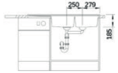
Ön Görünüm / Front View
