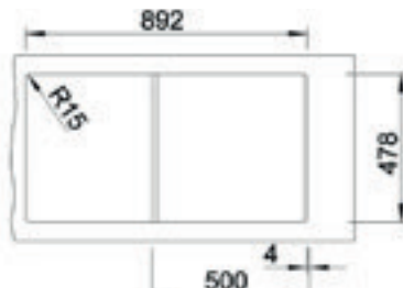
Tezgah Kesim Ölçüleri / Cut-Out
