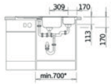
Ön Görünüm / Front View
