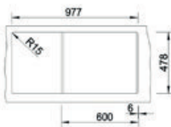
Tezgah Kesim Ölçüleri / Cut-Out
