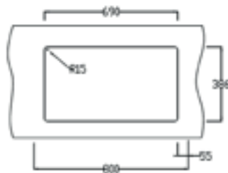
Tezgah Kesim Ölçüleri / Cut-Out
