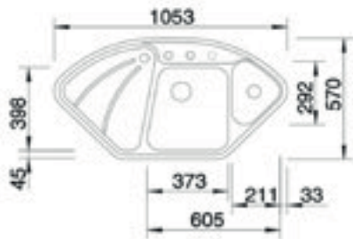
Üstten Görünüm / Top View
