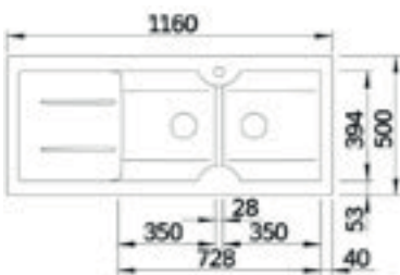
Üstten Görünüm / Top View
