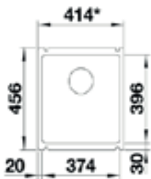
Üstten Görünüm / Top View
