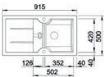
Üstten Görünüm / Top View
