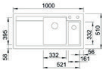
Üstten Görünüm / Top View
