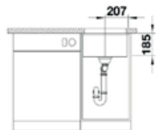
Ön Görünüm / Front View
