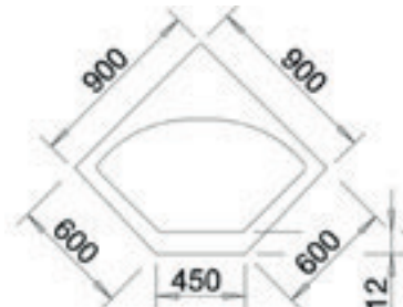
Tezgah Kesim Ölçüleri / Cut-Out
