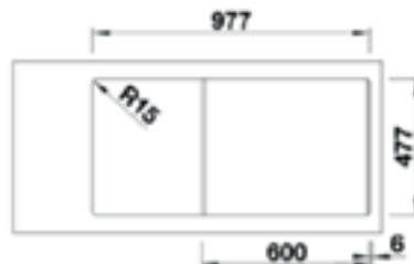
Tezgah Kesim Ölçüleri / Cut-Out
