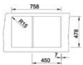
Tezgah Kesim Ölçüleri / Cut-Out
