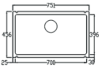
Üstten Görünüm / Top View
