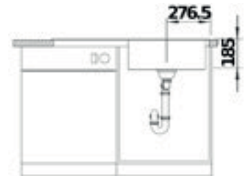
Ön Görünüm / Front View
