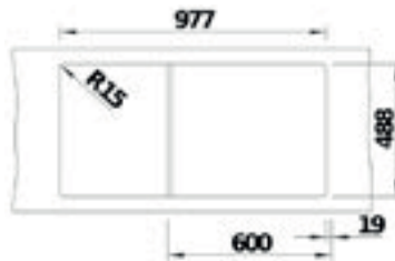
Tezgah Kesim Ölçüleri / Cut-Out
