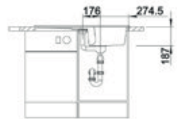
Ön Görünüm / Front View
