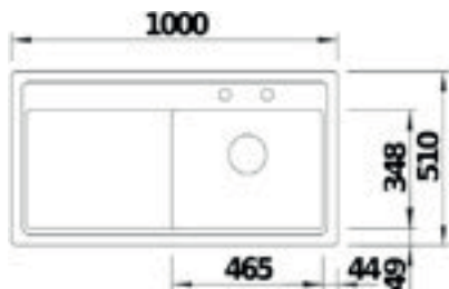
Üstten Görünüm / Top View
