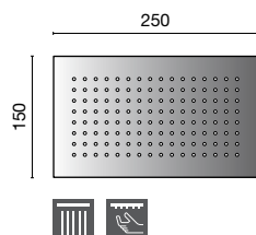
Rociador Recto 25x15 cm., con rótula. Recto 25 x 15 rain shower head, with ball joint.
