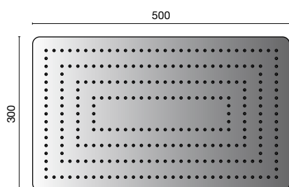
Rociador Recto 50x30 cm., sin rótula.
