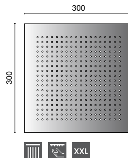
Rociador Square 30 cm., con rótula. Square 30 cm rain shower head, with ball joint.
