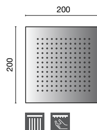
Rociador Square 20 cm., con rótula. Square 20 cm rain shower head, with ball joint.
