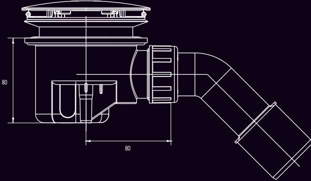
Viega Tekne Sifon Seti
