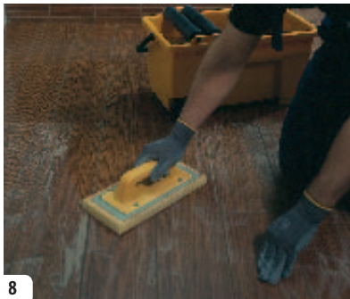
8- Limpiamos con un limpiador el resto de juntas que nos ha quedado.
