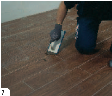
7- Rejuntado de la cerámica con el ancho aconsejado, aditivando con cl-stuk.
